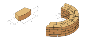
RD.3 Radial stretcher
