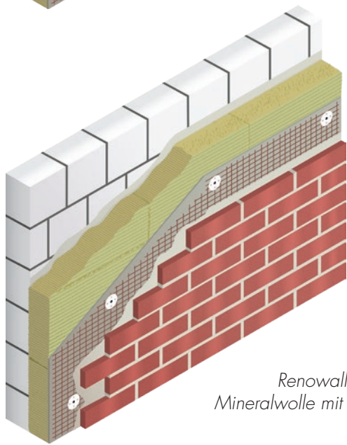
Renowall Fireproof System Mineralwolle mit hand- geformten Riemchen
